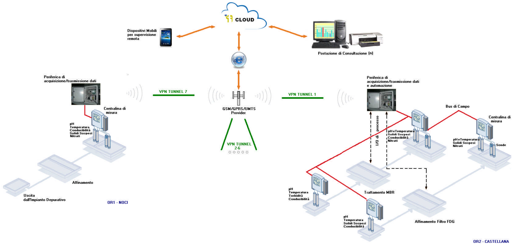
FIG.1 - Architettura Sistema di Telecontrollo PON IN.TE.R.R.A. in CLOUD
